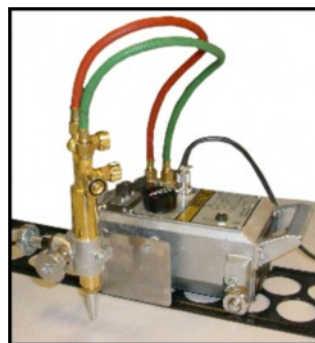
Barra para cortar círculos, Cortes de 38-2450mm (1½ - 96 in) de diametro.
