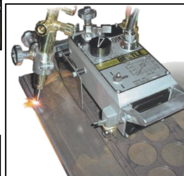
Barra para cortar círculos, Cortes de 38-2450mm (1½ - 96 in) de diametro.
